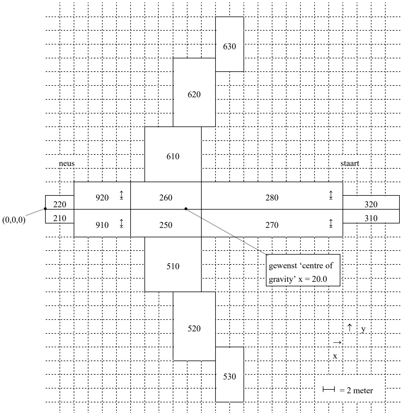
Figuur 7: bovenste niveau van het vliegtuigmodel voor de validatie
