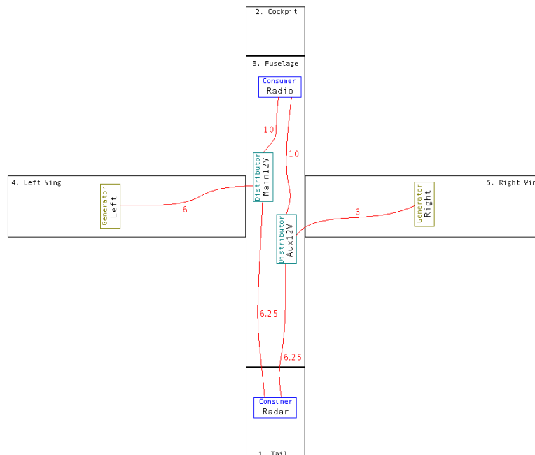
Figuur 1: een voorbeeld van een bekabelingschema 3
