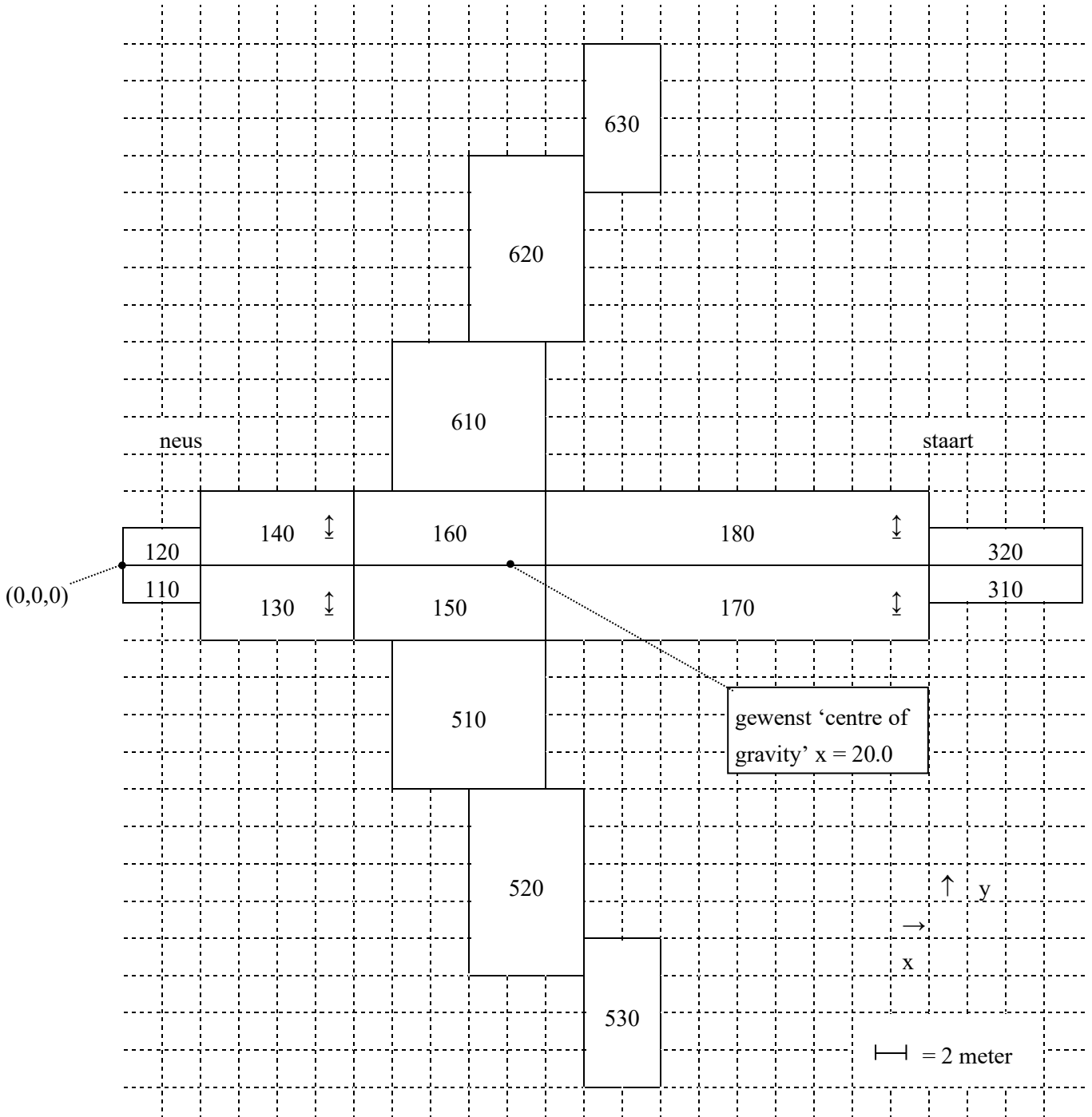
Figuur 6: onderste niveau van het vliegtuigmodel voor de validatie
